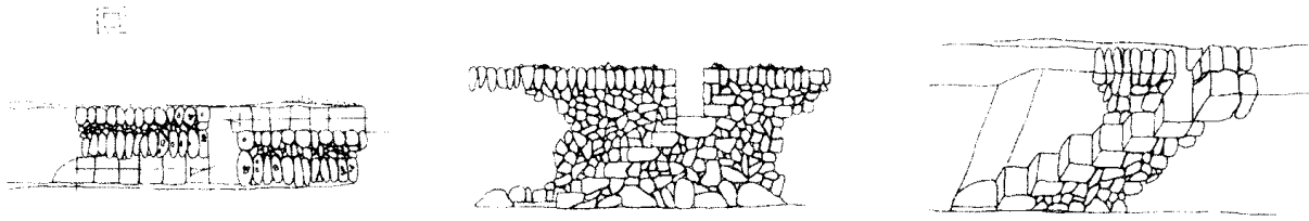
SCALA INCASSATA DI UN PARIETE DI TERRAZZAMENTO
