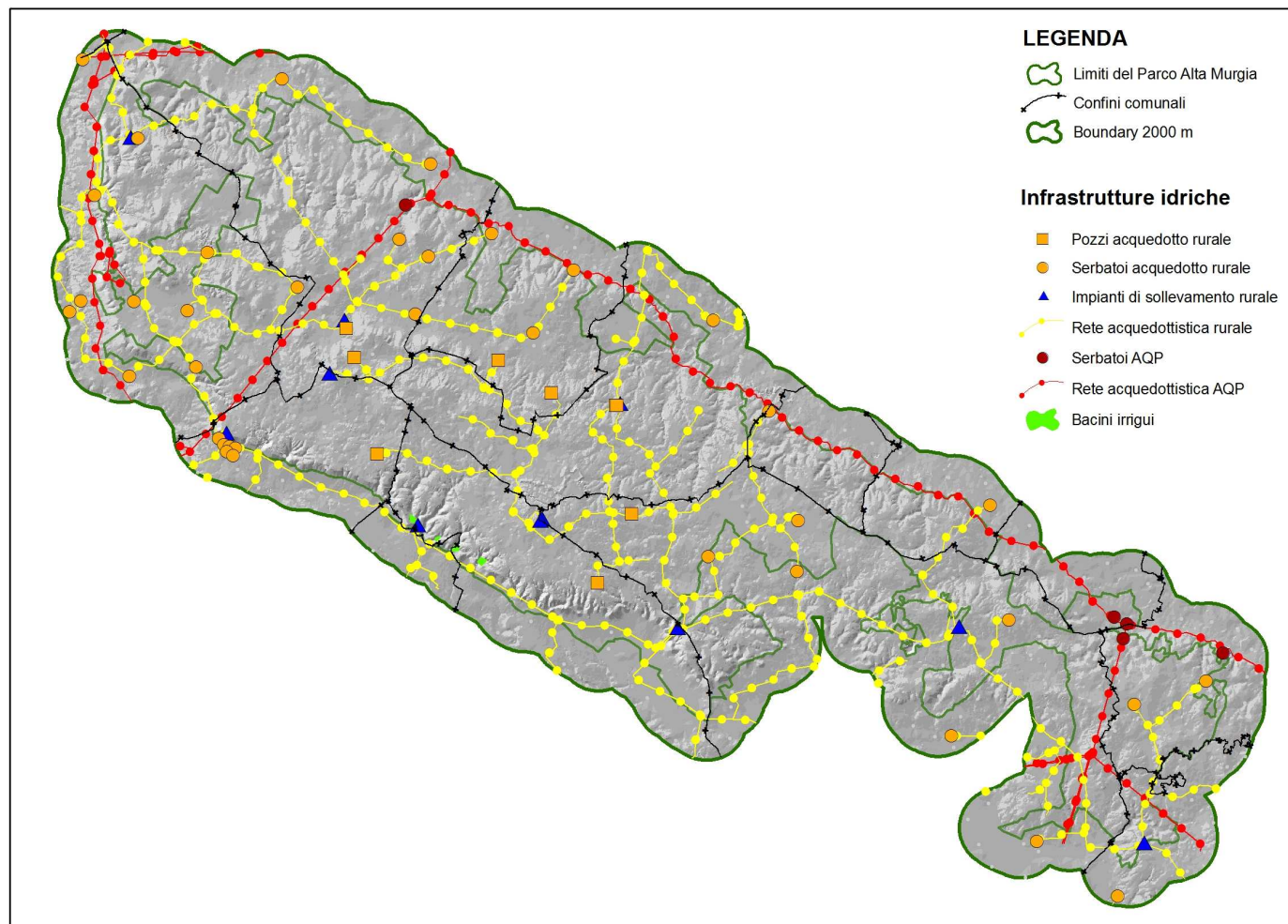
Figura 4-43 – Infrastrutture idriche.
