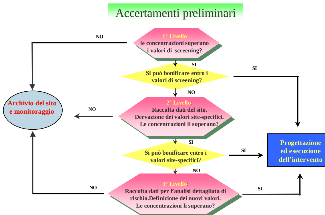
Figura 4-39 – Procedura RBCA.
